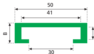
Profilo C - verde B=12 mm A= 6,5mm - (19080V) B=14 mm A= 8,5mm - (19053V) B=16 mm A=10,5mm - (19081V)
