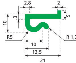
Profilo ZK (19007N - nero) (19007V - verde)
