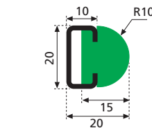
Profilo GB - verde (19035 - con profilo metallico inox) (19046 - con profilo metallico zincato)
