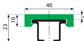
Profilo PIATTO (19063 con profilo metallico inox) (19063VC - verde) (19063NC - nero)
