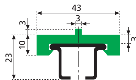
Profilo T (19064 con profilo metallico inox) (19064KVC - verde) (19064KNC - nero)
