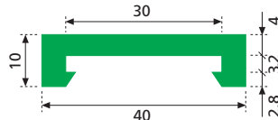
Profilo C - verde (19070)
