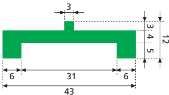
Profilo T rinforzato (19006N - nero) (19006V - verde)
