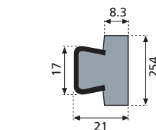
Profilo PIATTO - bianco (19031 con profilo metallico inox)
