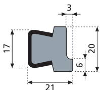
Profilo CON DENTE (19063 - con profilo metallico inox colore nero) (19063W - colore bianco)
